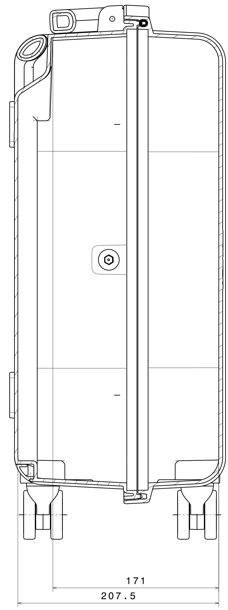
Schnittansicht A-A
